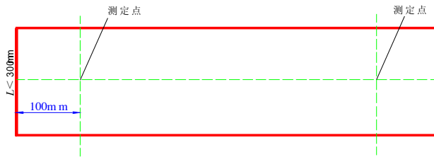
图 B.0.1-2 表面应力测量点示意
